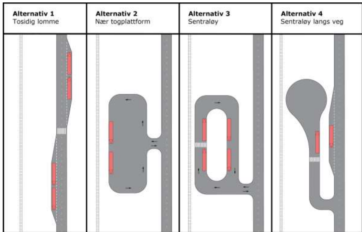
Figur 26 – Prinsippskisse av ulike uformingsvalg av bussbetjening av Hønefoss stasjon
